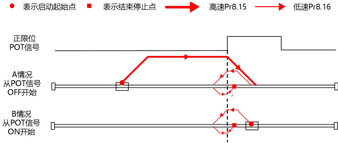
正限位回零路径图
