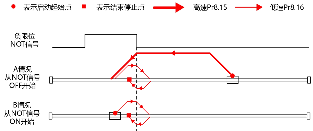
负限位回零路径图
